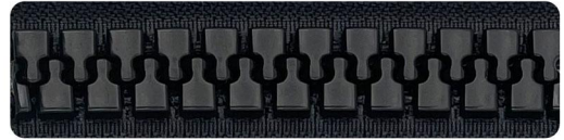
▲ 42 树脂 15# 普通牙 (坦克牙) 15# Plastic Tank Teeth
